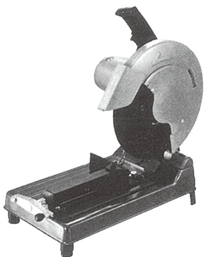
●高速カッター 2412N
