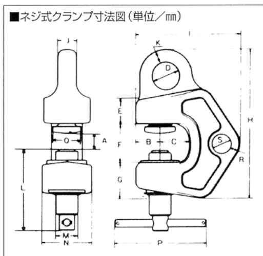
■ネジ式クランプ(全方向吊上げ)
