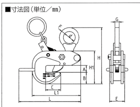
■横つり用クランプ
