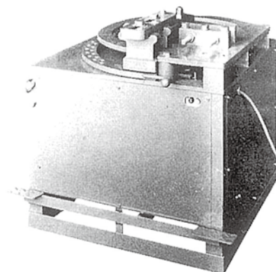
●鉄筋曲げ機 B-25
