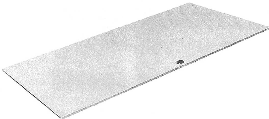
■鋼板／ゴムマット・寸法と重量
