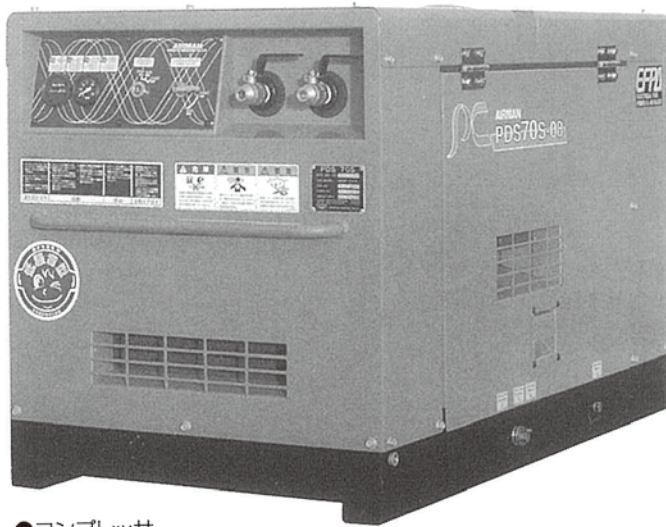
●コンプレッサー PDS-70S
