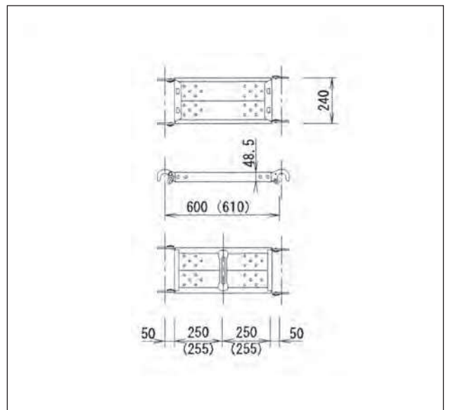
●鋼製布枠 2060 重量:3.72kg
