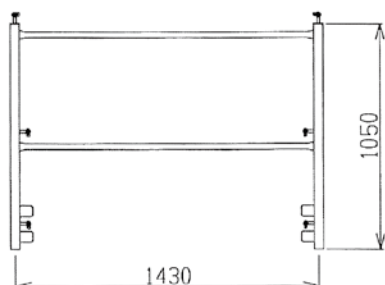
③ハンガーステージ手摺枠
