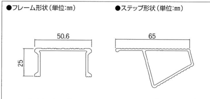
■アルミ合金製脚立仕様表
